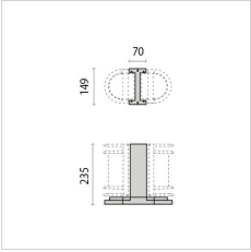
000404 Post 21 H200
