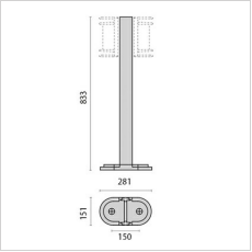
000412 Post 21 H800
